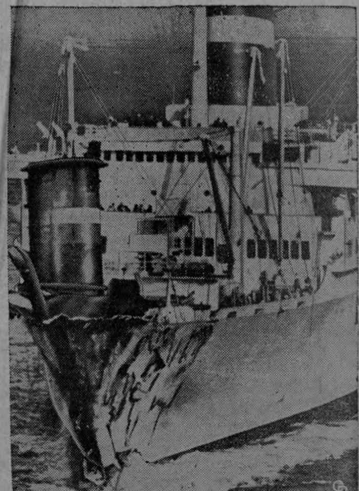
TRANSATLANTICO CHOCA CON BUQUE TANQUE.—Una chimenea del buque tanque Valchem quedó parada en la proa del lujoso transatlántico "Santa Rosa", después que los dos barcos chocaron a 30 millas de Atlantic City, N. J. Un marino del buque murió de las lesiones sufridas. El Santa Rosa, que costó $25,000,000 utilizó sus propias máquinas para regresar al puerto de Nueva York después que fue extinguida una conflagración en su cuarto de pinturas. Llevaba 512 personas, incluyendo 247 pasajeros.
