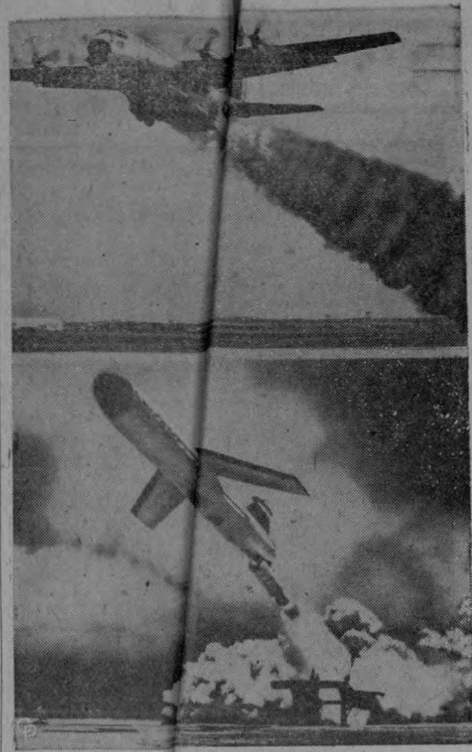
FUERTE EMPUJON AL AIRE.—Ayudado por ocho cohetes JATO, el nuevo C-130B Hércules de la Lockheed, con un peso máximo de 135.000 libras, despega de la Base Aérea de Eglin, en Florida. La ayuda con cohetes para el despegue es una serie de pruebas respecto a la fuerza de arranque de las hélices. El avión transporte de tropas, con una velocidad de 350 millas por hora, es fabricado para el Mando Táctico Aéreo. (Abajo) Un TM-76B Mace parte en una misión de entrenamiento en la base aérea de Holloman en Nuevo México. El TM-76A reemplazará a los cohetes Mador esta primavera. Los Matador están emplazados en Alemania Occidental.
