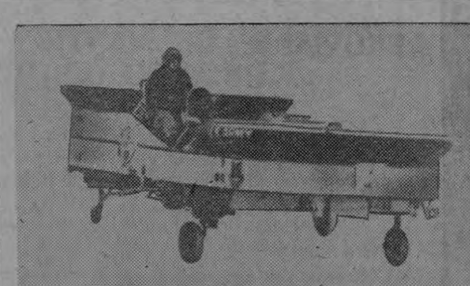
JEEP AEREO.—El VZ8P, vehículo terrestre-aéreo, sin alas, del ejército, está siendo probado en la Piasecki Aircraft Corporation, de Filadelfia, Pa. El VZ8P, que tiene completa maniobrabilidad en tierra, obtiene su poder de ascensión por medio de dos pequeños motores con hélices situados dentro de su estructura. Se informa que el vehículo es capaz de viajar rápidamente por las carreteras y entonces volar sobre los puentes que han sido destruidos.
